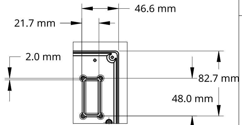
DETALLE C SCALE 1:3
