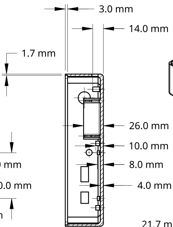
SECCIÓN B - B SCALE 1:3
